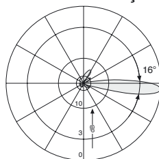
Diagrama Vertical 0°-14° downtilt elétrico
