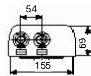
Vista inferior
