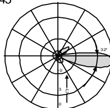
Diagrama Vertical 3° Downtilt elétrico
