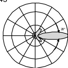
Diagrama Vertical 0° Downtilt elétrico
