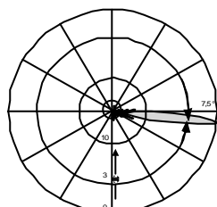
Diagrama Vertical 0,5° - 7° Downtilt elétrico ajustável
