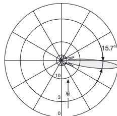
Diagrama Vertical 6°downtilt eléctrico
