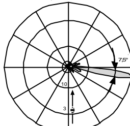
Diagrama Vertical 0° - 7° downtilt eléctrico
