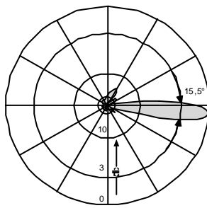
Diagrama Vertical 0° - 14° Downtilt eléctrico ajustable
