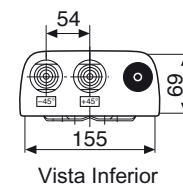
Vista Inferior
