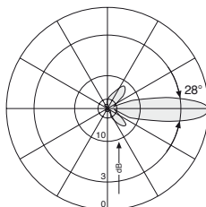
Diagrama Vertical 0°downtilt eléctrico
