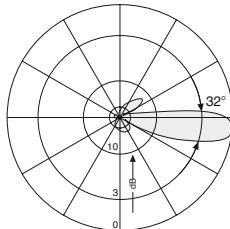
Diagrama Vertical 3° downtilt eléctrico
