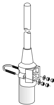
Montaje en el tope
