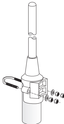
Montagem no topo do mastro
