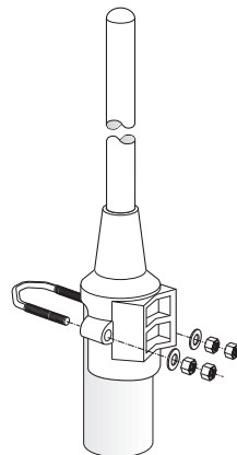
Montagem no topo do mastro
