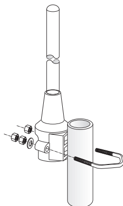
Montagem Lateral
