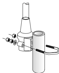
Montagem Lateral no Mastro
